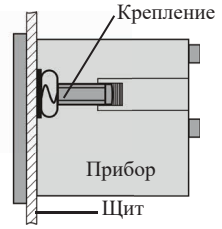
Рис. 2 – Установка прибора
