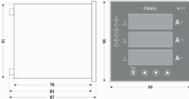
Рис. 3 – Размеры прибора
